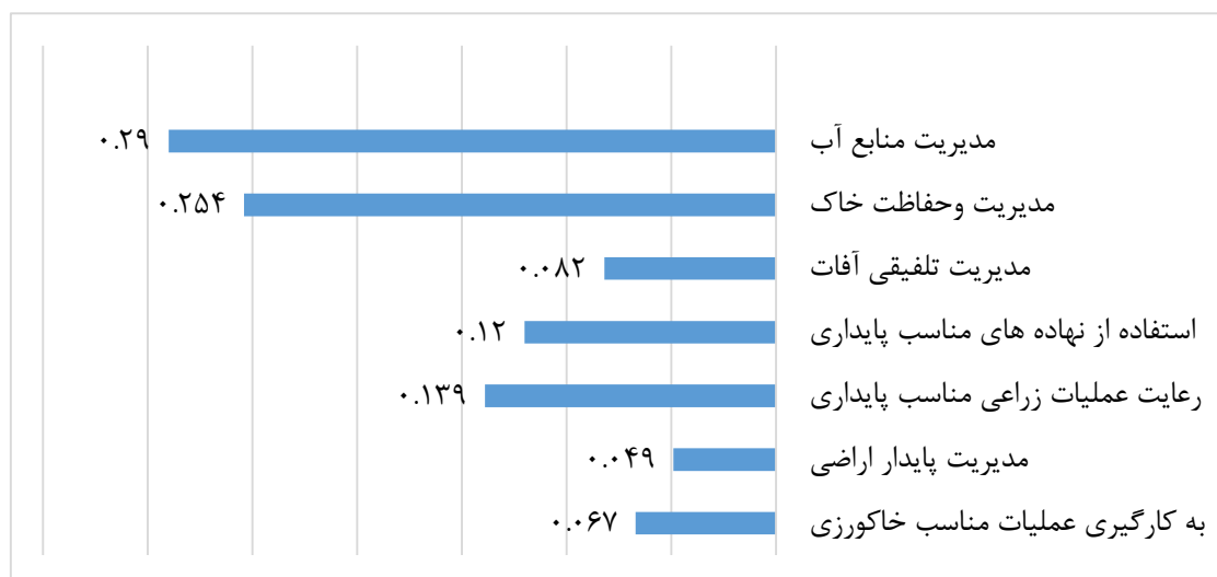
شکل ۵- نمودار وزن مولفه های شاخص اکولوژیکی
